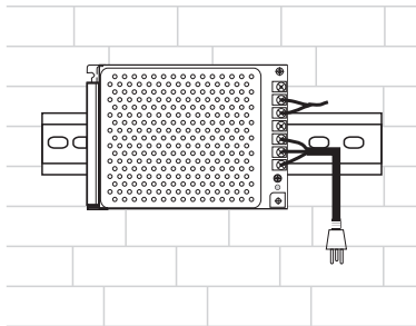
DIN rail mounting
